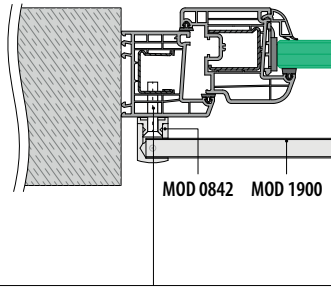
Rahmenmontage
