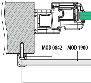
Fassadenmontage
