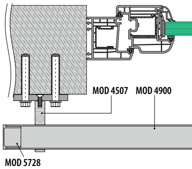
Fassadenmontage
