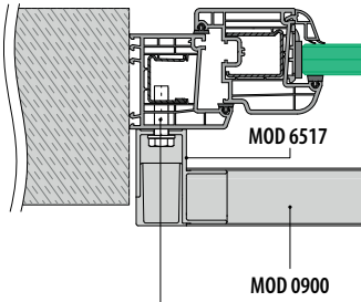
Rahmenmontage
